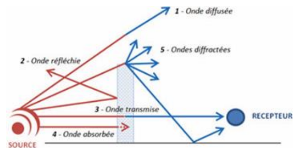
Phénomènes intervenant dans la propagation du bruit
