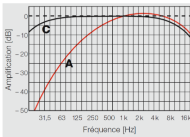
Courbes de pondération A et C
